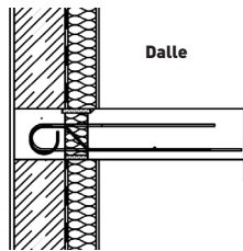
Jonction dalle-facade en ITI
