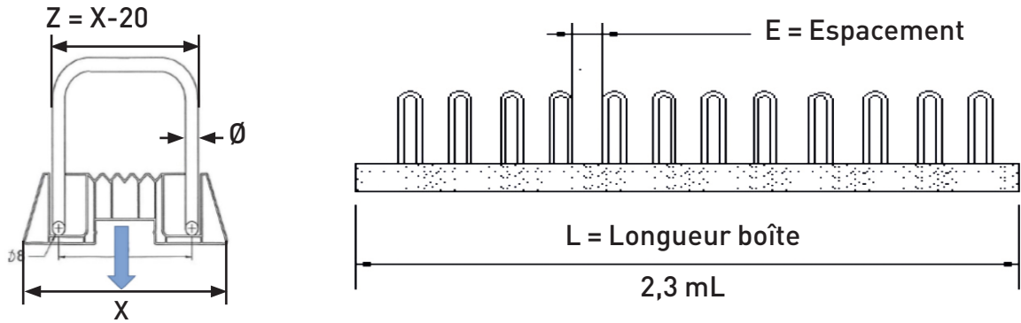
Système d'engravure pour aimant de fixation
