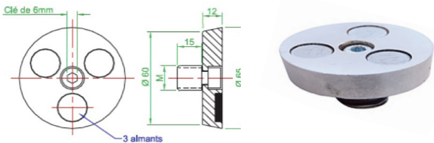
Dimensions des flasques acier magnétiques
