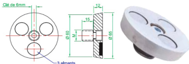
Dimensions des flasques acier magnétiques
