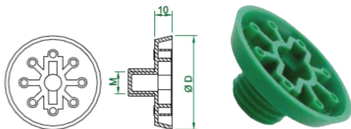
Dimensions des flasques PVC rondes
